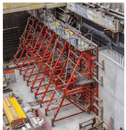
Die nötigen Arbeitsbühnen sind entsprechend an dem jeweiligen Schalungssystem angebracht.
