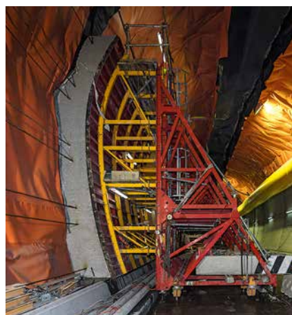
Beim einhäutigen Betonieren leitet der Stützbock die hohen Lasten an die Fundamente ab.
