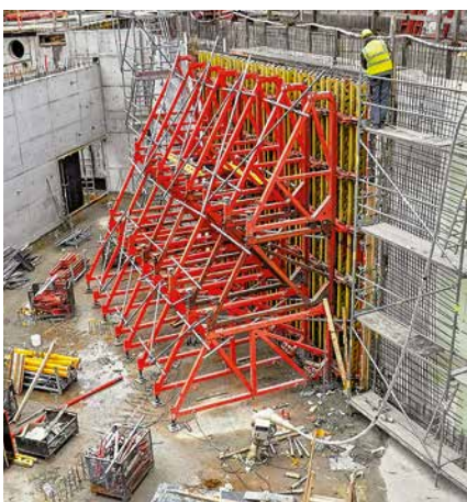
An jeder Stelle des Stützbocks SB-A0, A, B, C ist die Kräfteinleitung gewährleistet.
