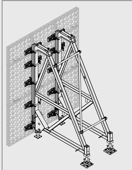
Die Stützbocke werden an Stellen von vertikalen Stößen der montierten Paneele am Ausgleichsriegel DUO befestigt.
